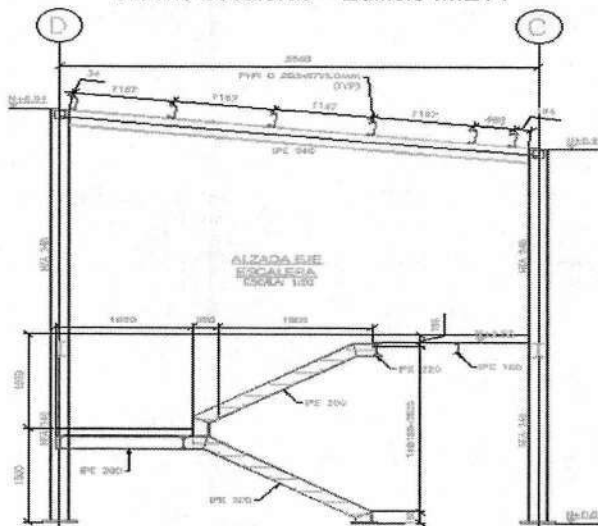
Figura No. 7. Diseño escaleras – Edificio IMETY
