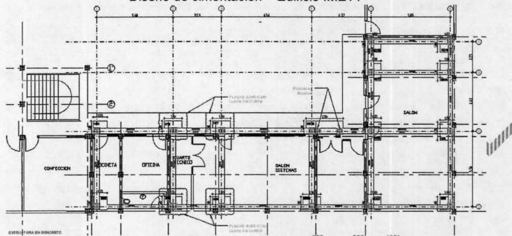
Figura No. 5. Diseño de cimentación – Edificio IMETY
